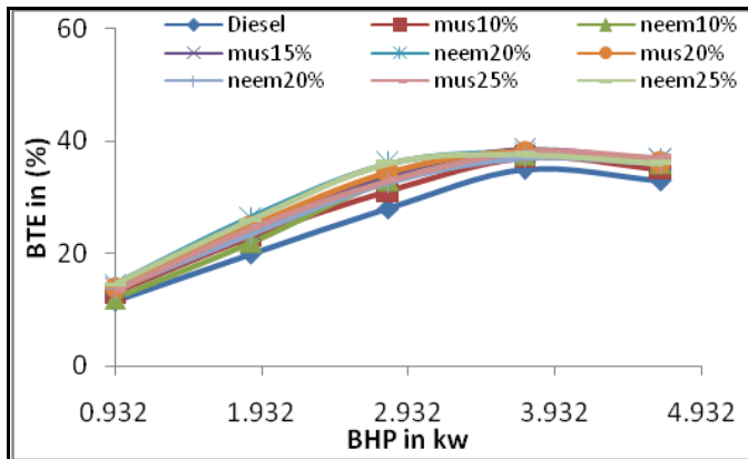
Figure-5. Bp Vs BTE
