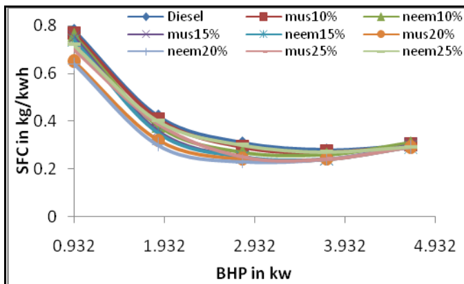
Figure-4. Bp Vs SFC
