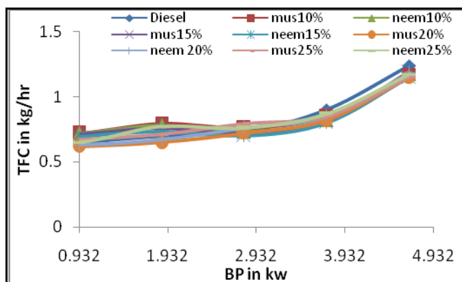
Figure-2. Bp Vs TFC
